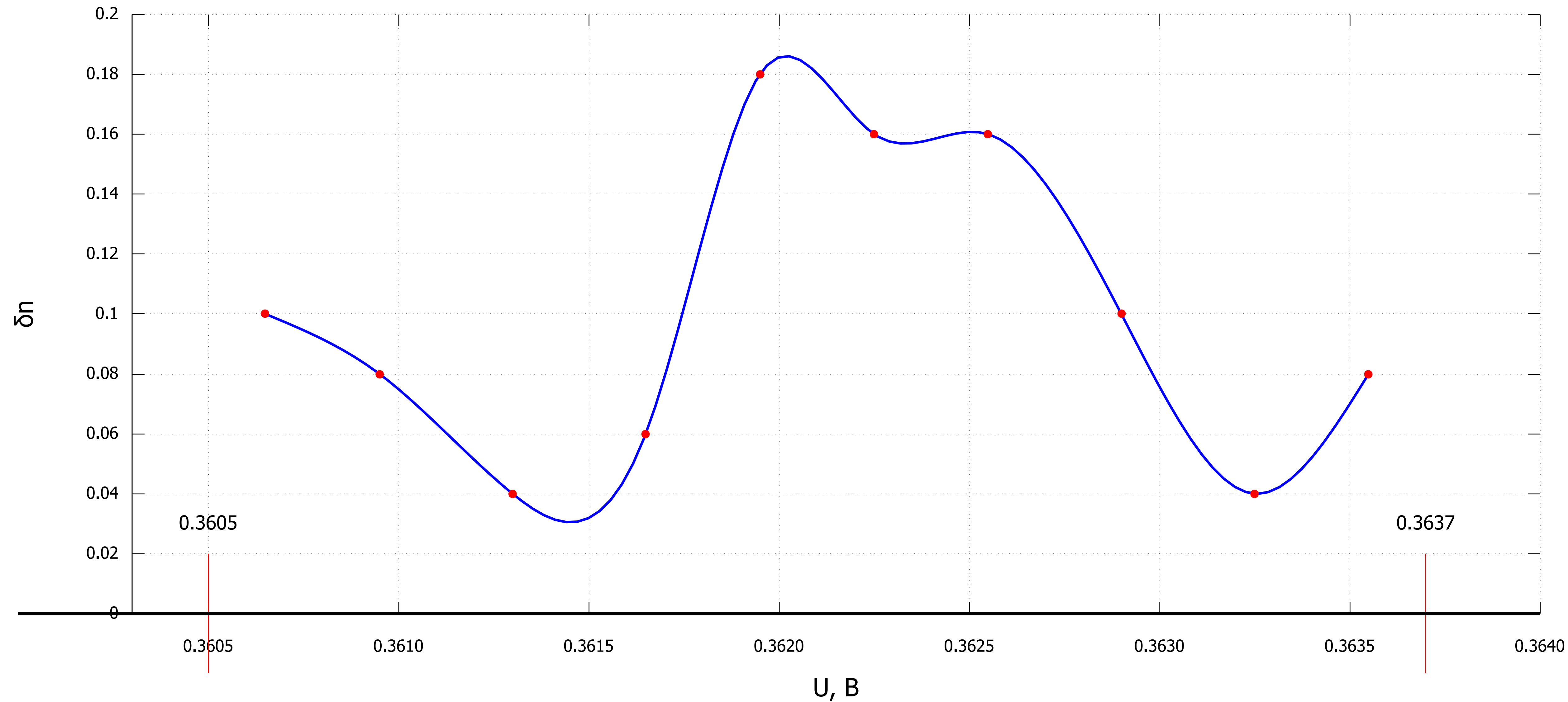
График распределения \delta n = f(U)
